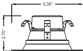
A-DL-10-27 / A-DL-10-30 / A-DL-10-50
